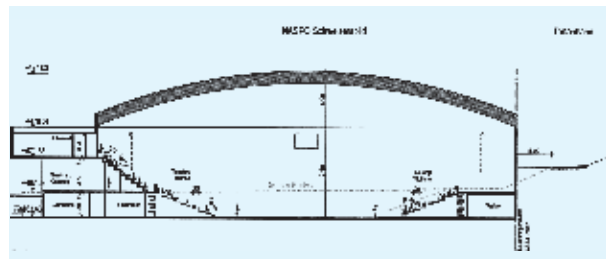
Querschnitt NaSpo-Halle mit angrenzender Tartanbahn des Schulhauses Gräfler
